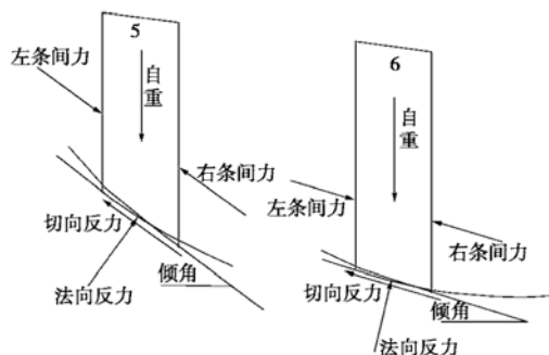
图1 瑞典条分法中的条间力示意图
