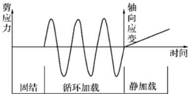
图 1 砂砾料液化后静力特性试验加载过程
