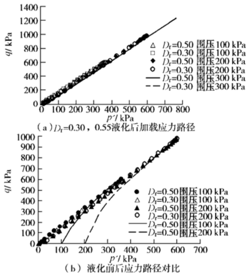
图 4 应力路径
