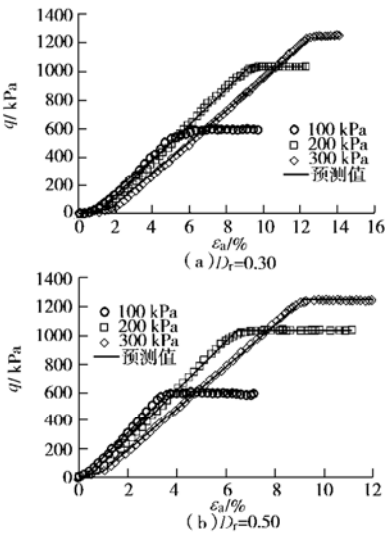
图 7 试验曲线与预测曲线
