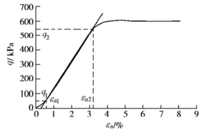
图 5 交点定义
