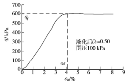
图 6 定义破坏应力、应变
