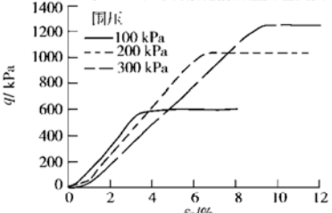
(b) D_r=0.50 砂砾料不同围压液化后应力应变关系
