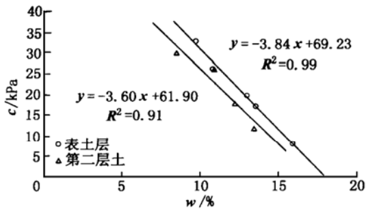
图8 粘聚力随含水率变化关系
