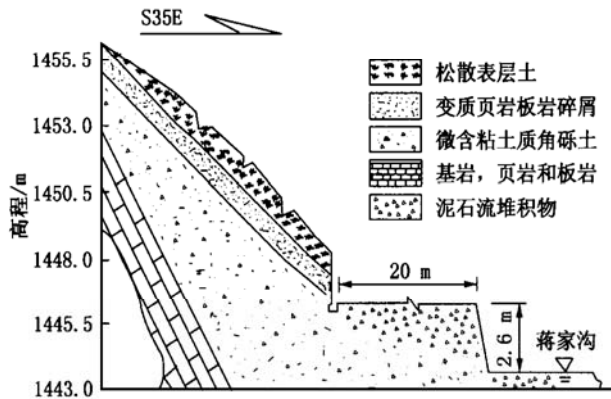
图1 试验斜坡剖面图
